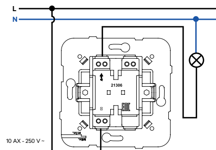
Interrupteur Rotatif
