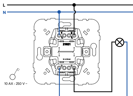
Interrupteur Bipolaire
