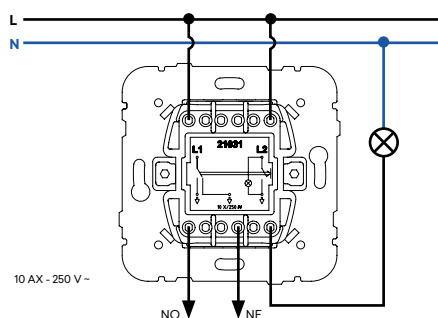
Interrupteur Card-system
