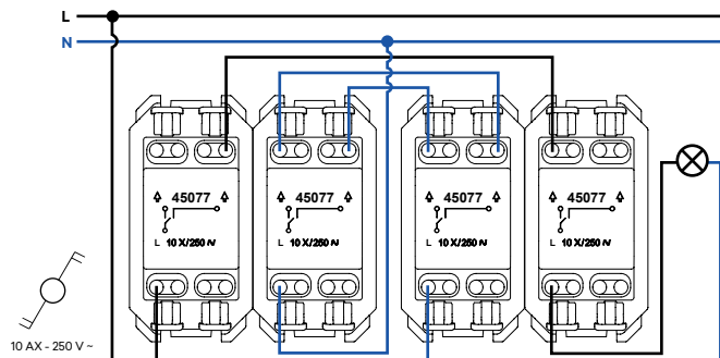
Va-et-Vient Bipolar
